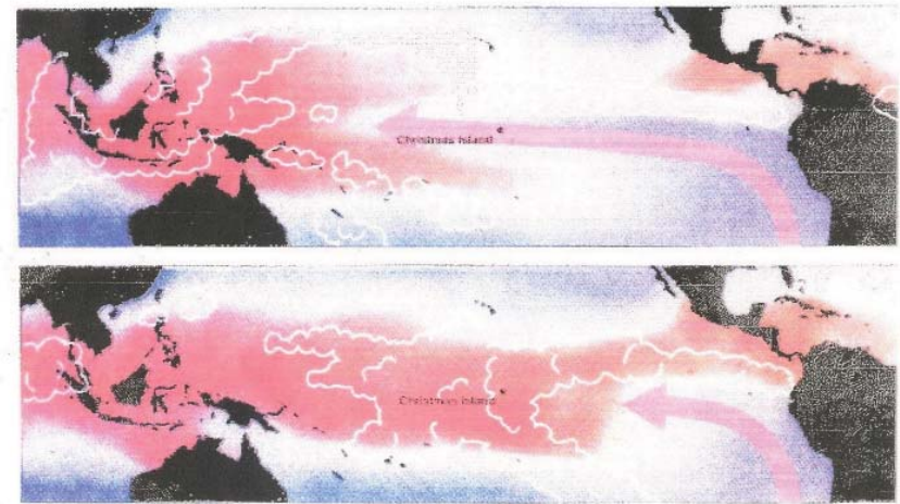
Figura 1. Movimiento de lluvias al Este durante EL Niño, indicado por las flechas en la figura inferior. La imagen superior muestra un movimiento de nubes normal.
