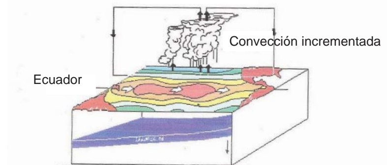
Figura 2. Condiciones que se presentan por la ausencia (arriba) o presencia (abajo) de El Niño.
