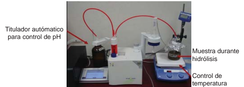
Figura 4. Sistema de hidrólisis, donde se observa el titulador automático que controla el pH de la solución y un sistema para el control de la temperatura.
