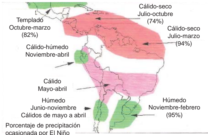
Figura 5. Potencial de impactos de El Niño.
