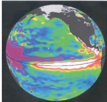
Figura 4. Imagen tomada por el satélite Topex-Poseidón, donde se observan las temperaturas de la superficie del mar.
