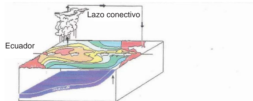
Figura 1. Movimiento de lluvias al Este durante EL Niño, indicado por las flechas en la figura inferior. La imagen superior muestra un movimiento de nubes normal.
